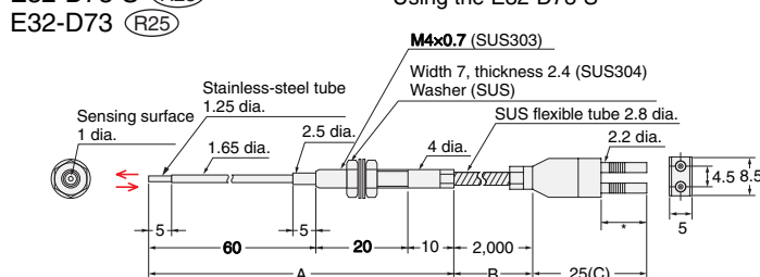
E32-D73-S (R25) Using the E32-D73-S
