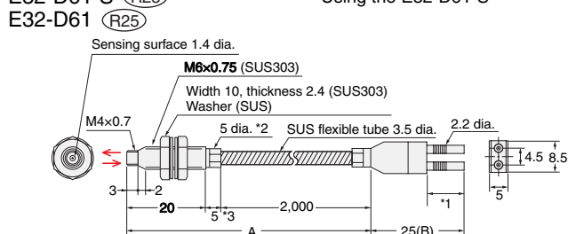
E32-D61-S (R25) Using the E32-D61-S
