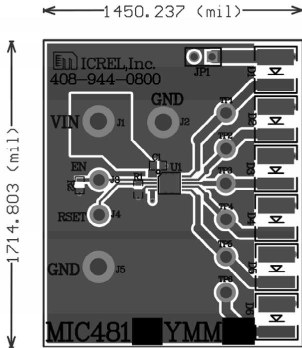
Top Layer
