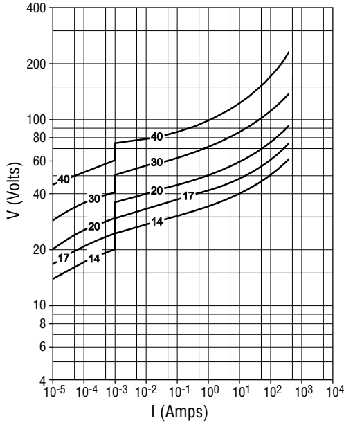
Model Size 1210 - (AV 14 K 1210 401 ~ AV 40 K 1210 401)
