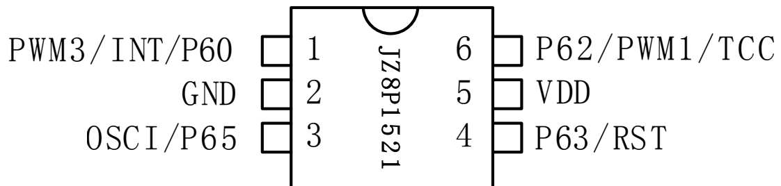
JZ8P1521-6PIN 脚位图
