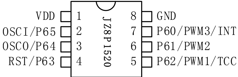
JZ8P1520-8PIN 脚位图
