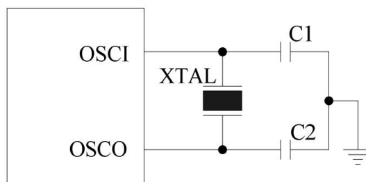
晶体/振荡器电路
