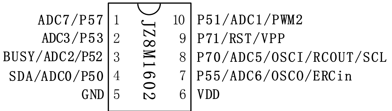
JZ8M1602-10PIN 脚位图
