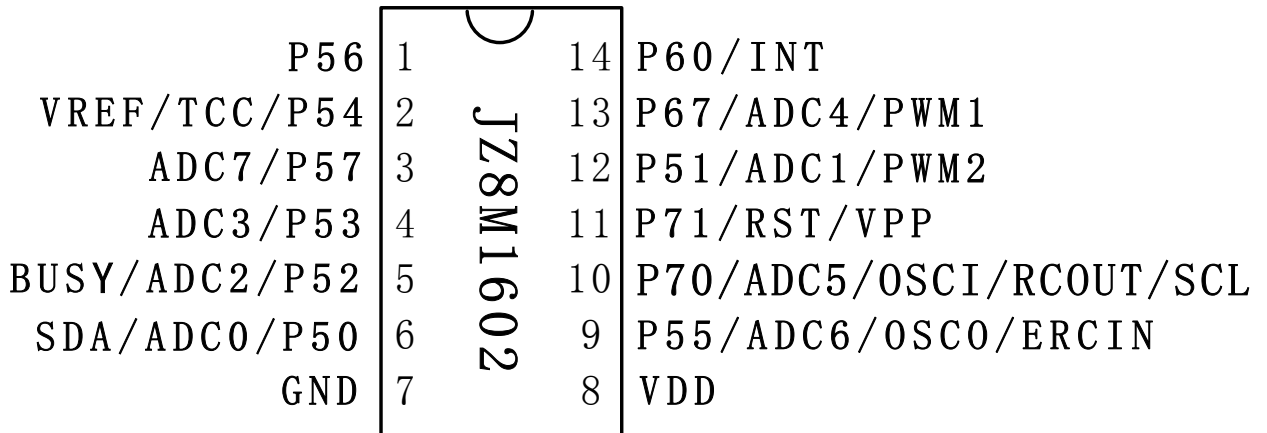
JZ8M1602-14PIN 脚位图
