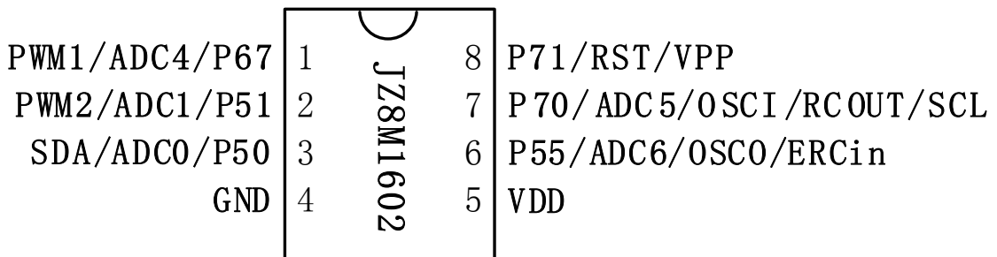
JZ8M1602-8PIN 脚位图
