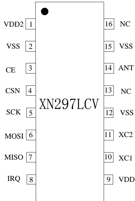
图5.2 XN297LCV芯片引脚功能图
