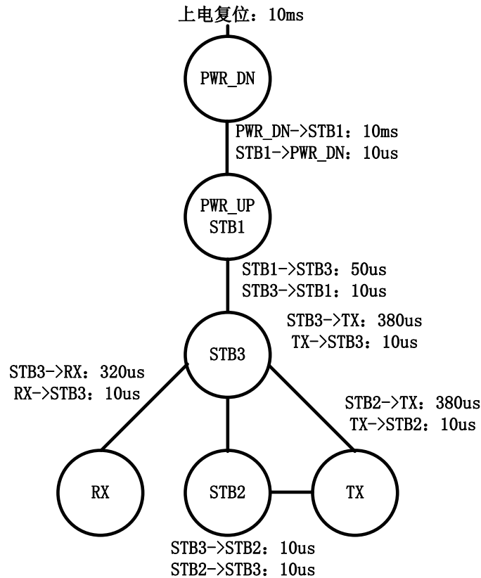
图6 工作状态图
