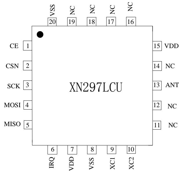
图5.1 XN297LCU芯片引脚功能图
