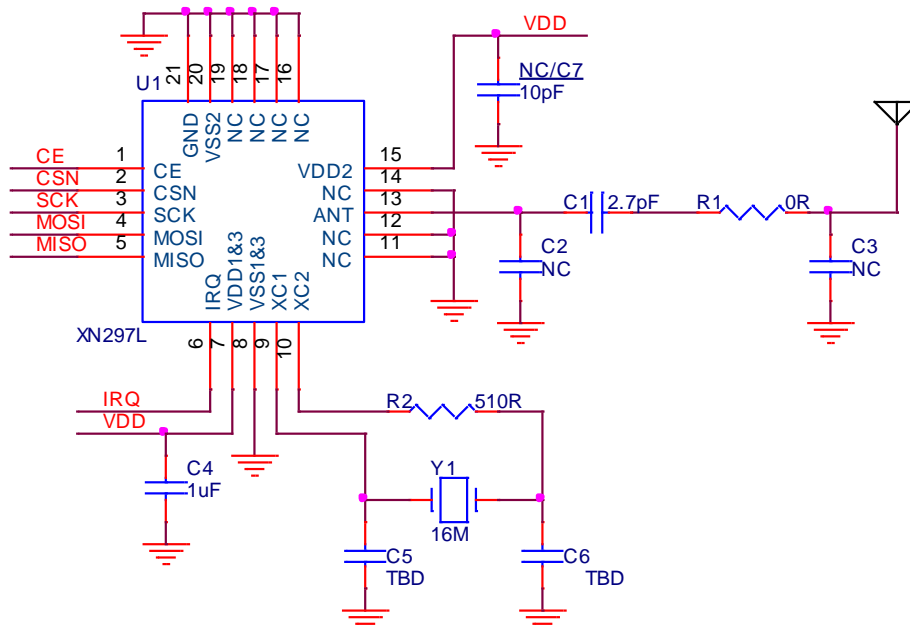
图11 XN297LCU的应用电路
