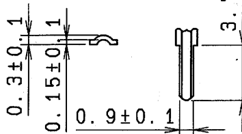
基板挿入部端子形状詳細(3:1) TERMINAL DETAIL
