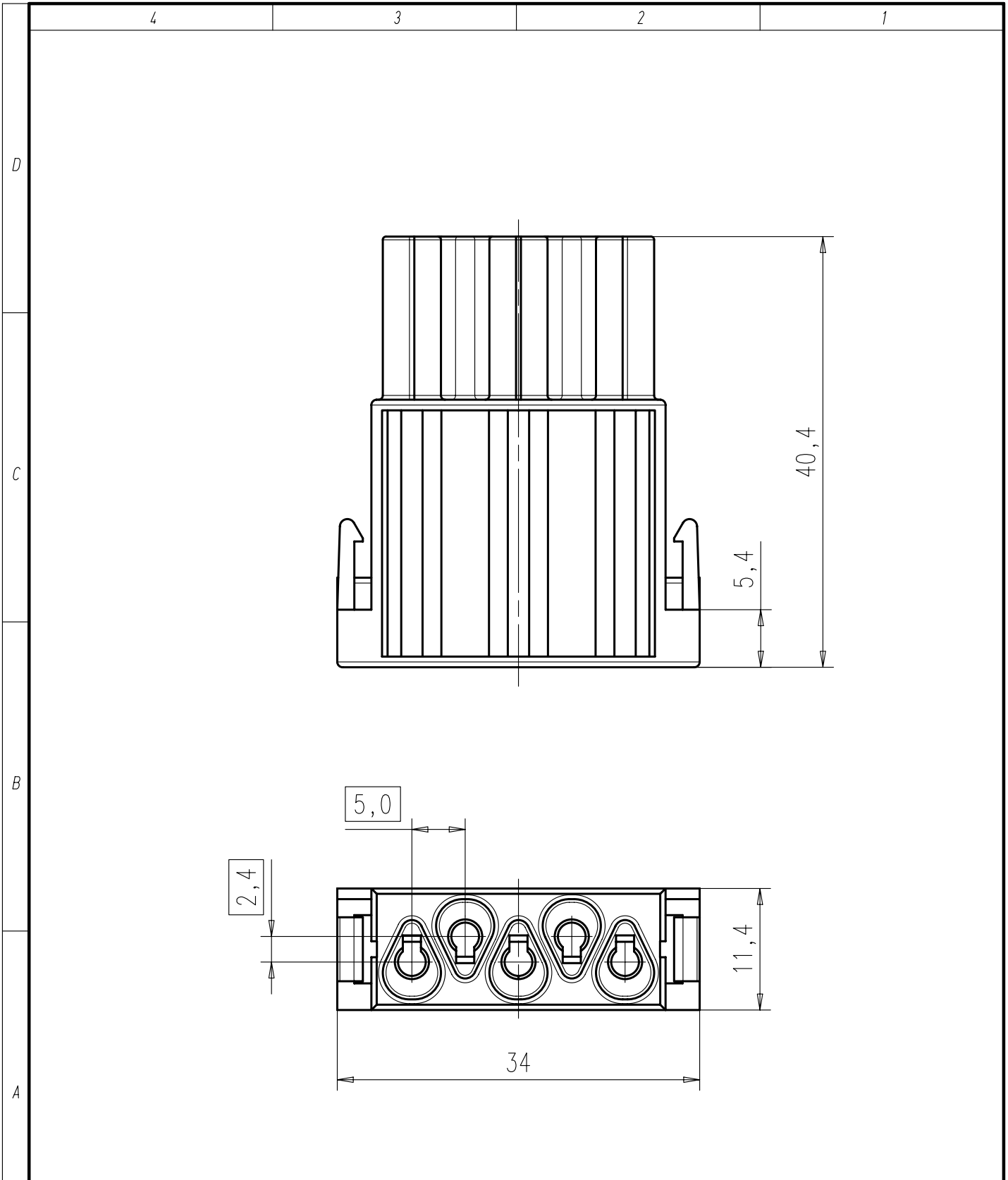
PE Kontakt 2mm voreilend
