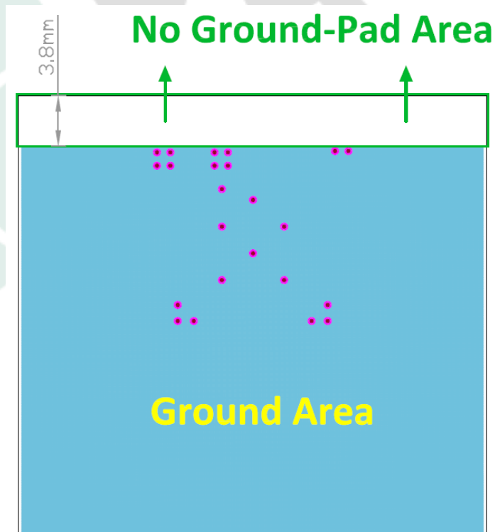
Bottom layer
