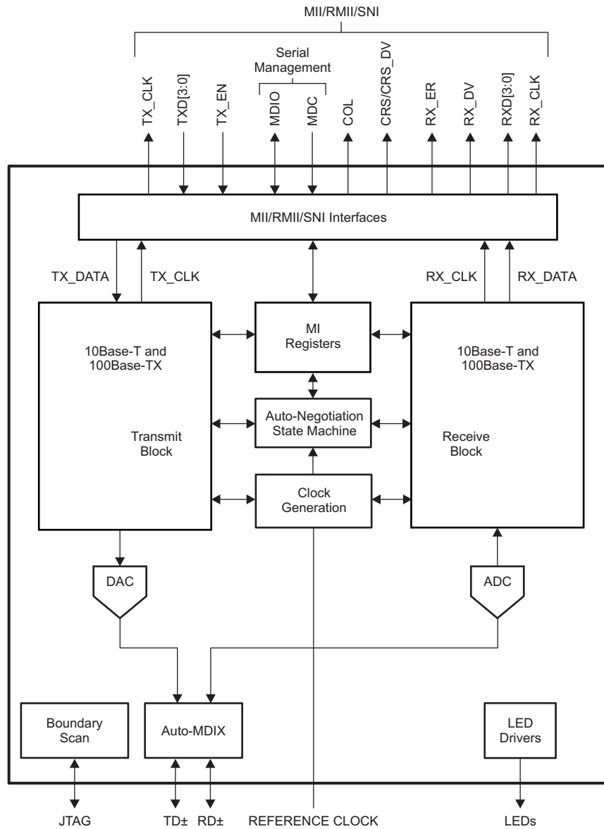
图 2-1. 器件方框图
