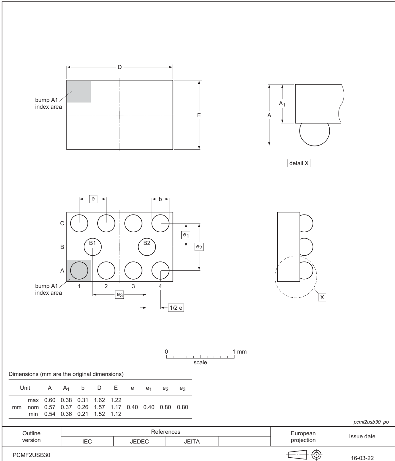
Fig 25. Package outline WLCSPP10
