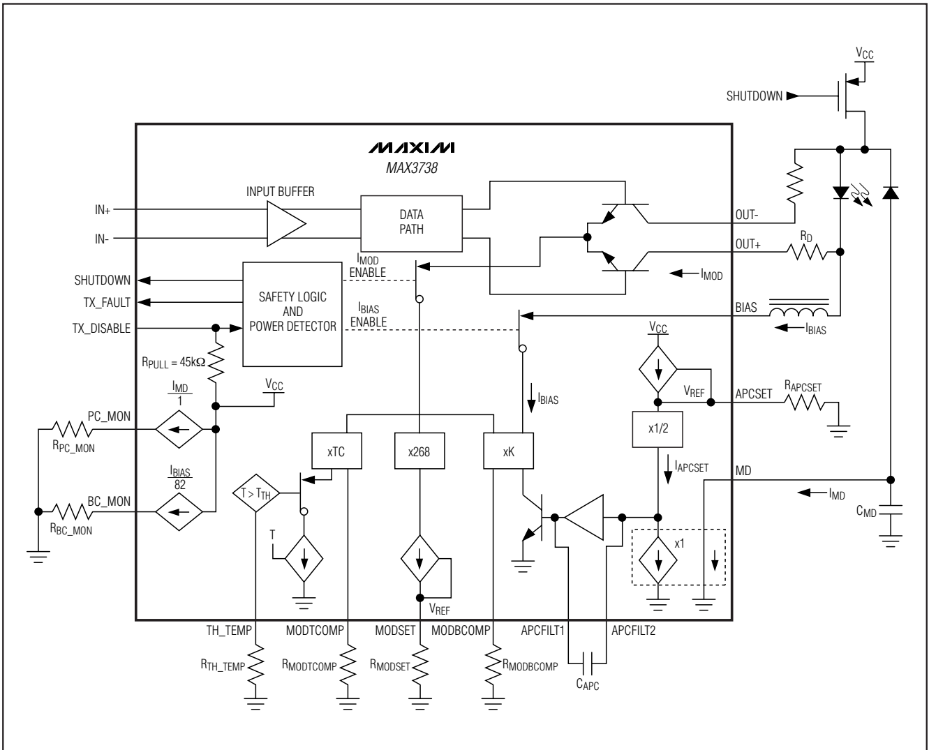
图4. 功能框图
