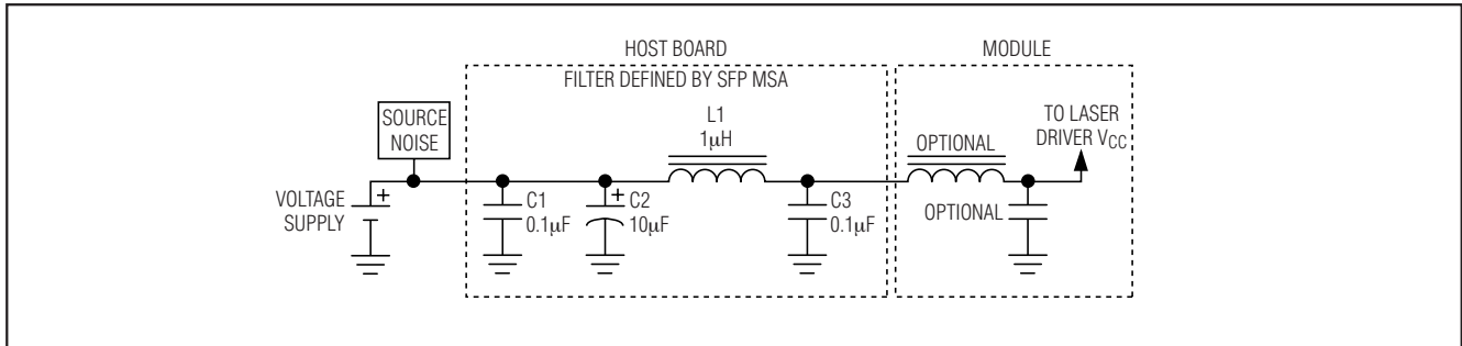
图3. 电源滤波器
