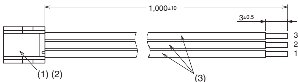
Wiring
