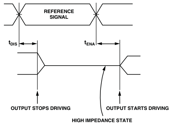
Figure 27. Output Enable/Disable
